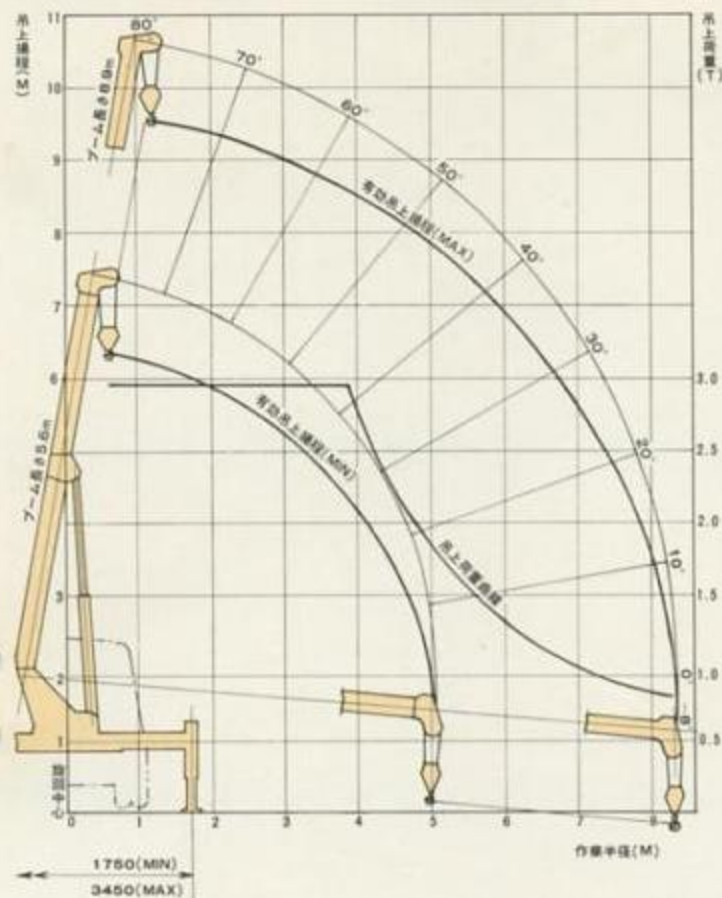
(1) D801(E)型クレーン車性能曲線図
