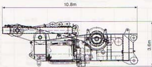
上部回転体（リア部）×1
